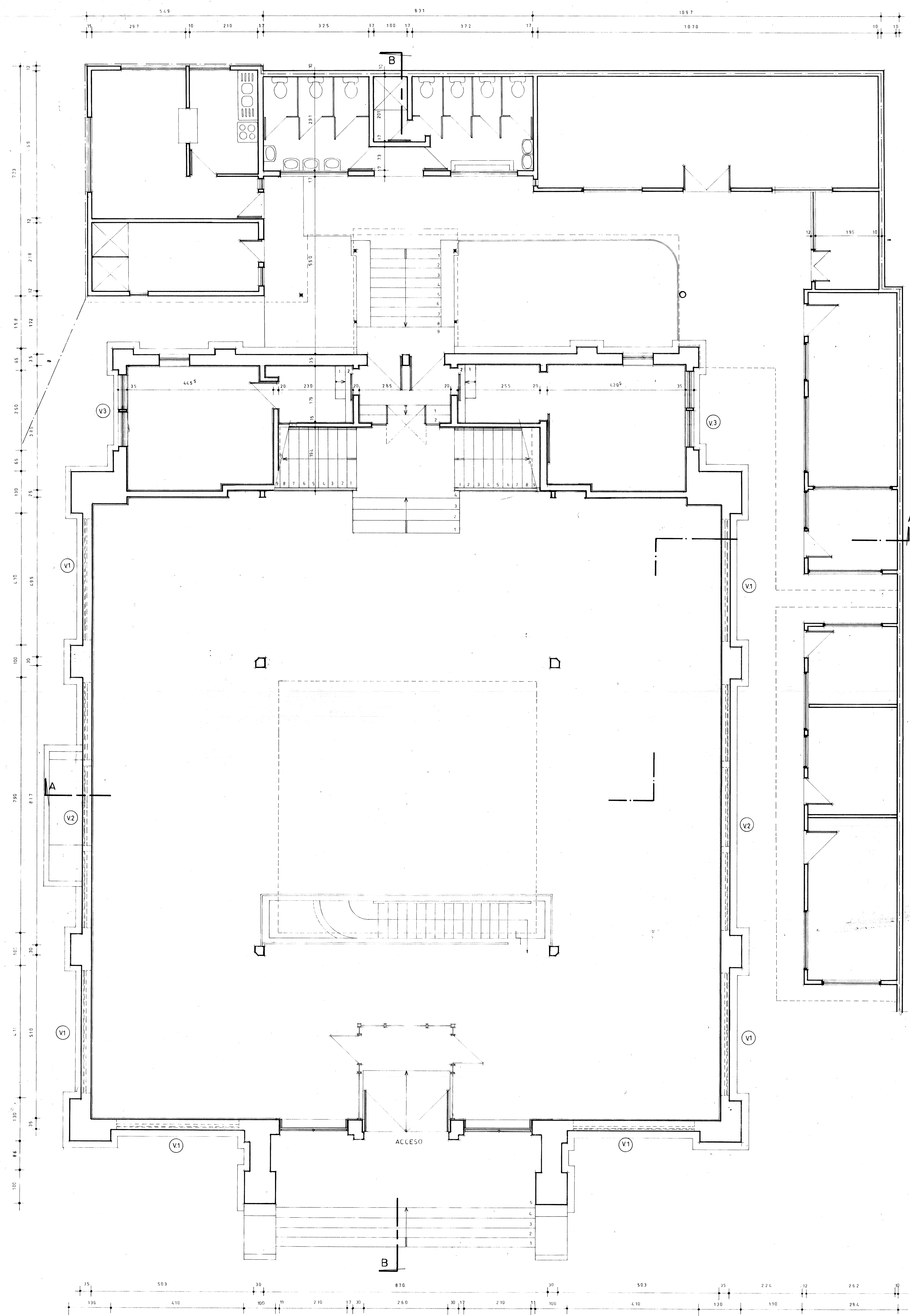
PLANTA 1º PISO 1:50
