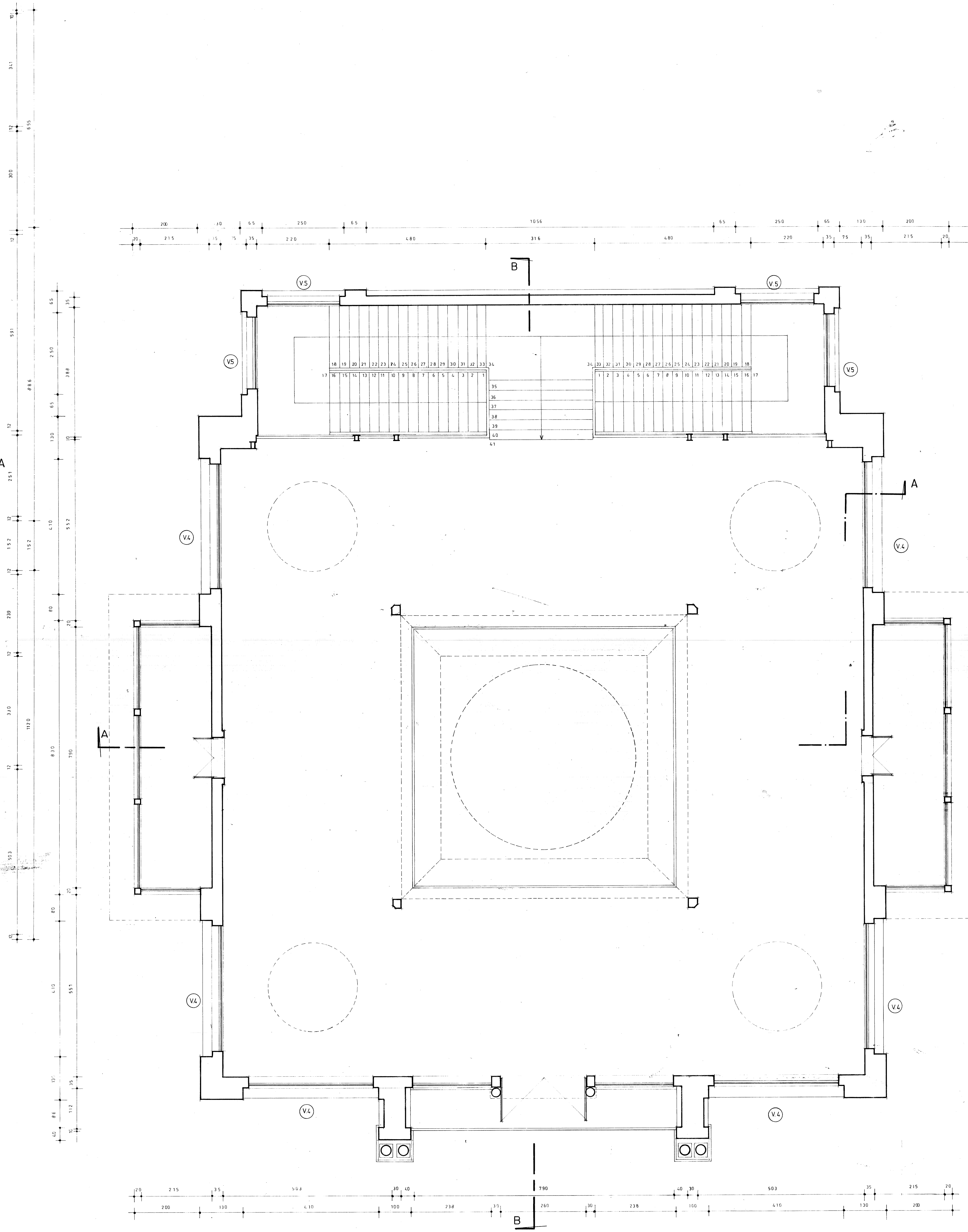
PLANTA 2º PISO 1:50
